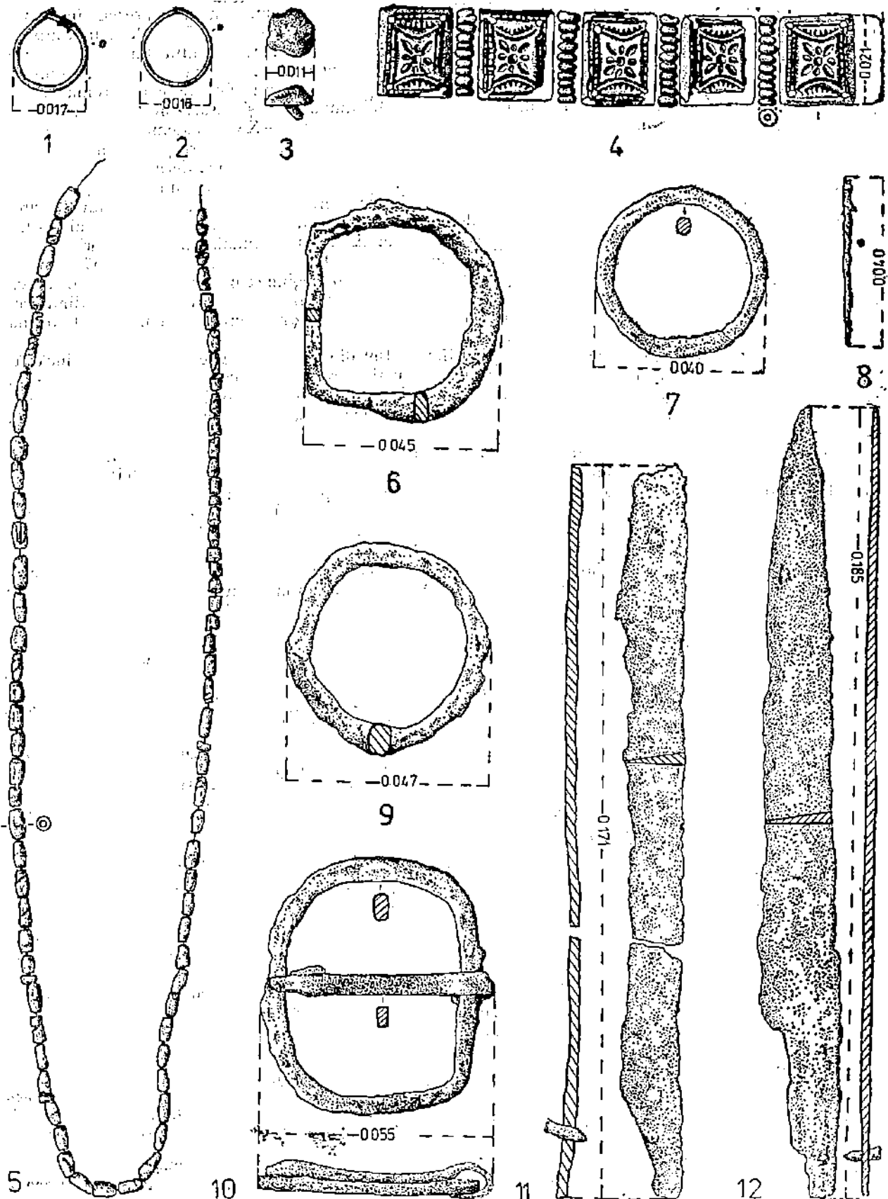
Fig. 5. Hudum. Cercei (1-2), șintă de la încălțăminte (3), plăcuțe și mărgelile de la diademă (4), șirag de mărgelile (5), catarame (6, 10), verigi de la centură (7, 9) ac de cusut (8), cușite (11-12) descoperite în mormintele 149 (1), 137 (2), 169 (3), 144 (4), 170 (5), 147 (6-7), 162 (8), 157 (9-11) și 158 (12) din necropolele 1 (137, 144, 147) și 2 (157, 158, 169, 170).
